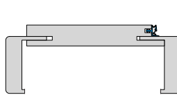
Futter rund FU-RF, 60 mm
