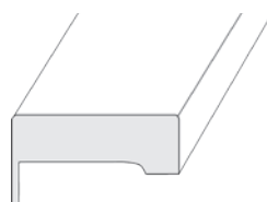
Zarge NC, 55 mm Kantenradius 2 mm
