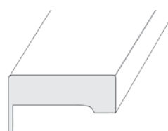
Zarge NC, 55 mm Kantenradius 2 mm
